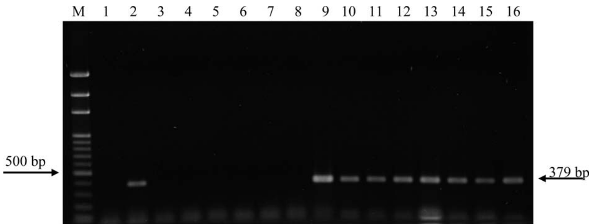
圖二、應用 PCR 技術以引子對 SfL1 / SfR2 鑑定莴苣細菌性葉腐病菌。M，100 bp DNA marker；1，negative control；2， Pseudomonas cichorii (芹菜葉斑病菌)；3， P. syringae pv. lachrymans (胡瓜角斑病菌)；4， P. syringae pv. phaseolicola (菜豆斑點病菌)；5， P. syringae pv. pisi (豌豆斑點病菌)；6， P. syringae pv. syringae (紫丁香花斑點病菌)；7， P. syringae pv. tabaci (菸草斑點病菌)；8， P. syringae pv. tomato (番茄葉斑病菌)；9，Sf 010 (向日葵細菌性葉斑病菌， P. cichorii )；10~16，Pc 1~7 (莴苣細菌性葉腐病菌， P. cichorii )。
